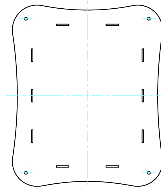
下カバー裏面 / Bottom cover Backside
